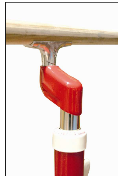
Liaison porte-mains / montants entièrement métallique avec protection intégrée
